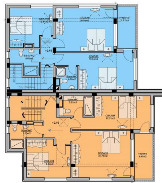
Чертеж: РАЗПРЕДЕЛЕНИЕ ВТОРИ ЕТАЖ
