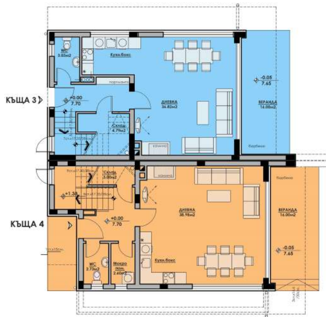
Чертеж: РАЗПРЕДЕЛЕНИЕ ПЪРВИ ЕТАЖ
