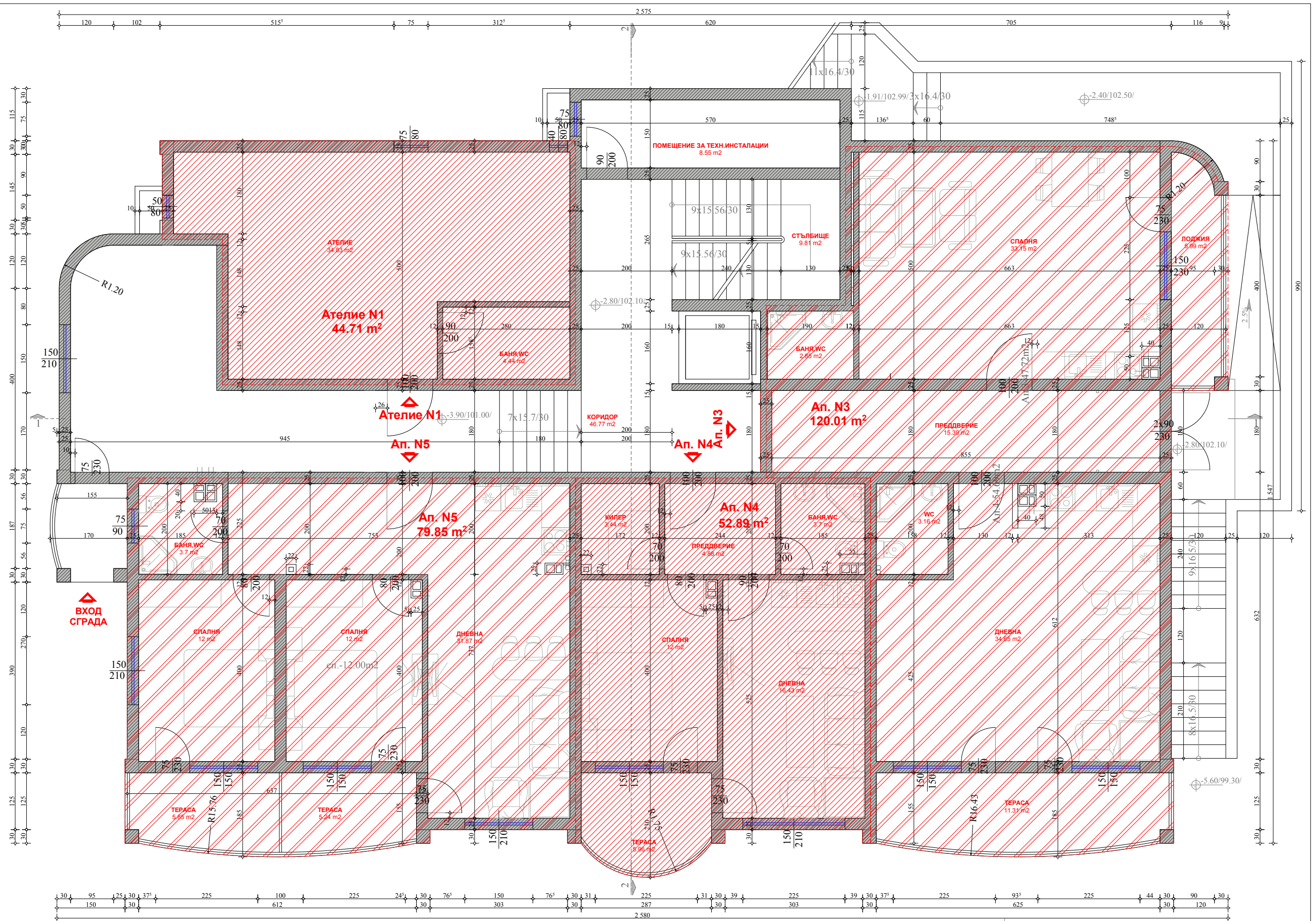
Разпределение на сутерен I - кота -2.80/102.10/ и -3.90/101.00/ - 381.58 m 2
